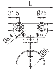
电缆滑车
