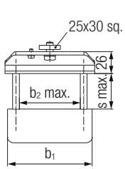
端部夹具
