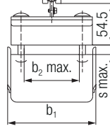
电缆滑车
