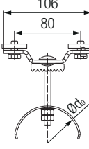
端部夹具
