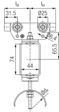
牵引滑车
