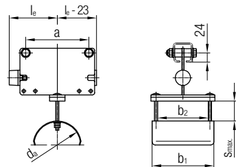
End Clamp 1)
