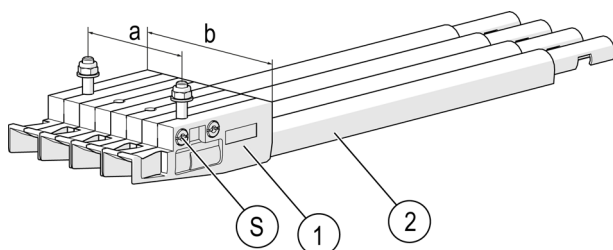
Fig. 46: End cap
