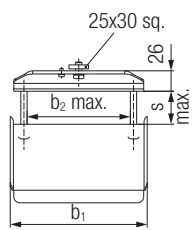
端部夹具
