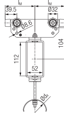
牵引滑车
