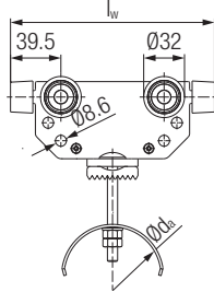
电缆滑车
