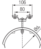
端部夹具
