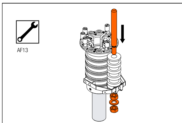
Fig. 16: Install the brush bolt.
