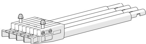
Fig. 18: End cap 081174
